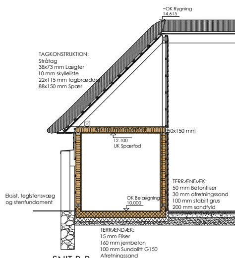
SNIT B-B
