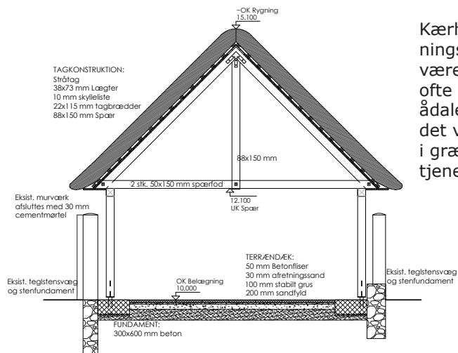
SNIT A-A
